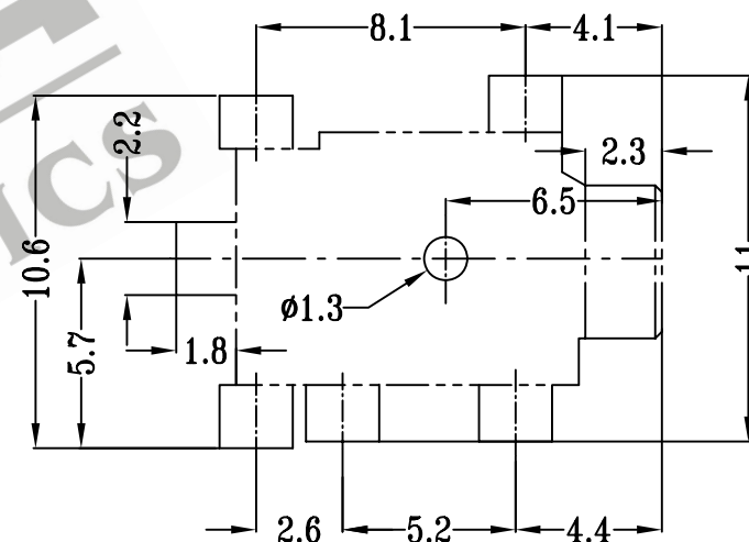
P.C.B LAYOUT
